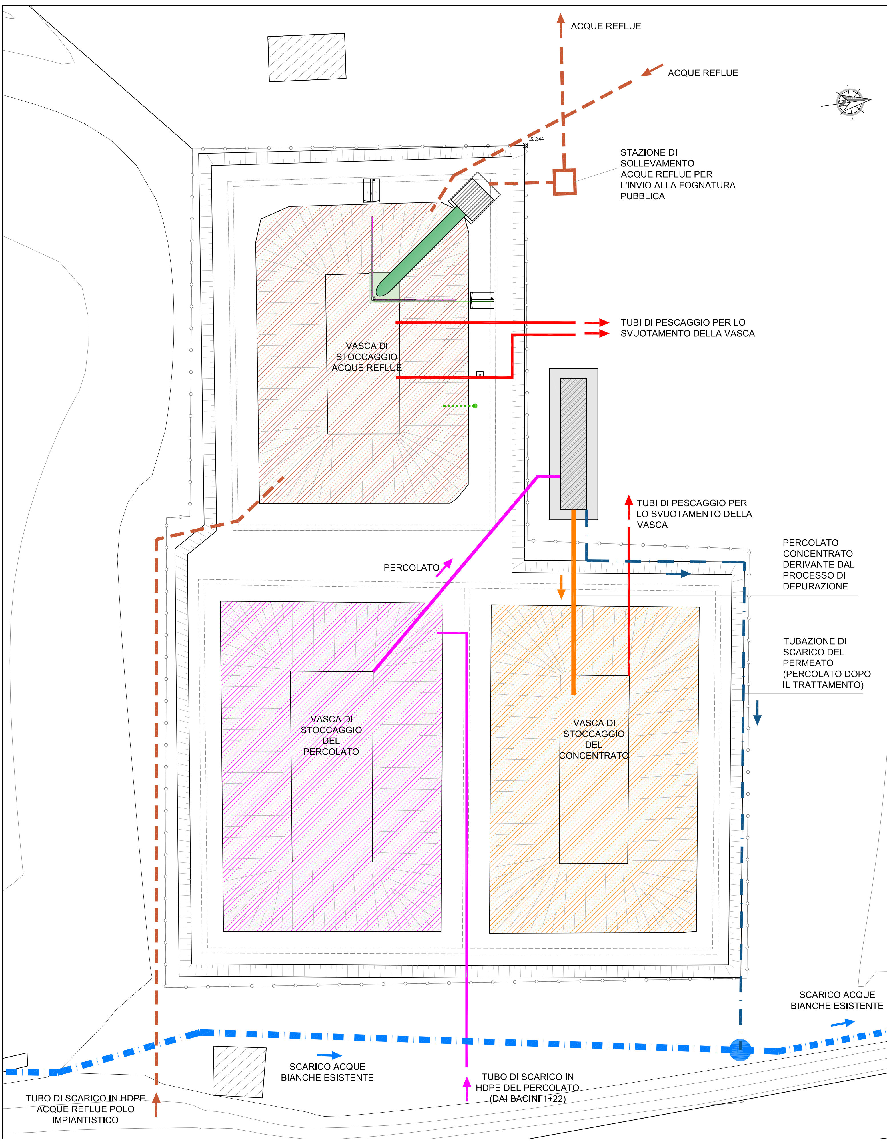
KEYPLAN - scala 1:5.000
